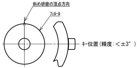
APC整端模式図
